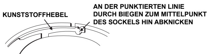
Abbildung 3b: Entfernen des Melders aus dem Meldersockel
