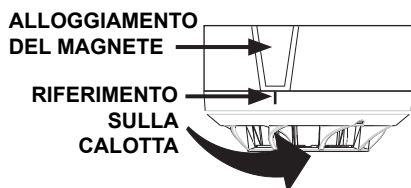
Figura 2: Montaggio del sensore sulla base
