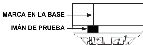
Figura 5: Posición del imán de prueba
