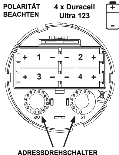
Abbildung 4: Batterieinstallation und Adressdreheschalter
