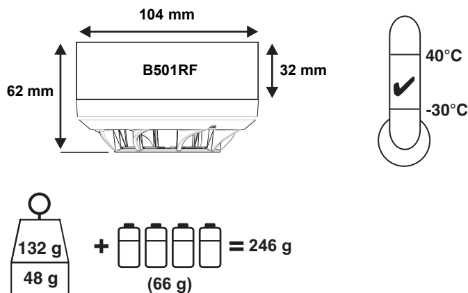
Figura 1: Montaggio B501RF
