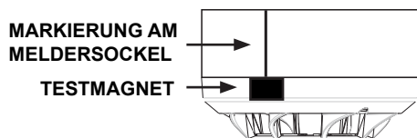
Abbildung 5: Position des Testmagneten
