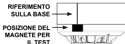
Figura 5: Posizione del magnete per il test
