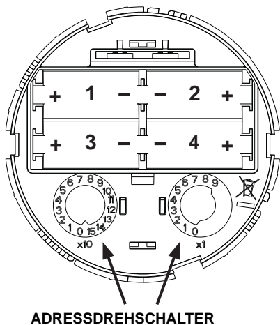
Abbildung 4: Batterieinstallation und Adressdrehesalter
